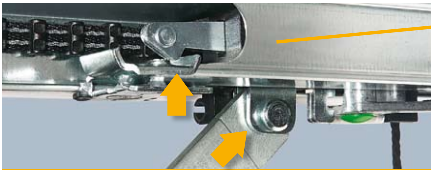
De deurvergrendeling in de aandrijvingsrail - een Hörmann-patent
