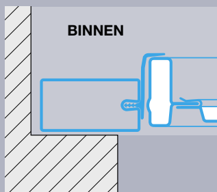
Deurtype N80 Aanslag achter de opening
