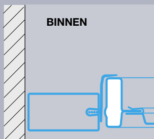
Deurtype N80 Aanslag in de opening
