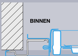
Deurtype F80 Aanslag vóór de opening
